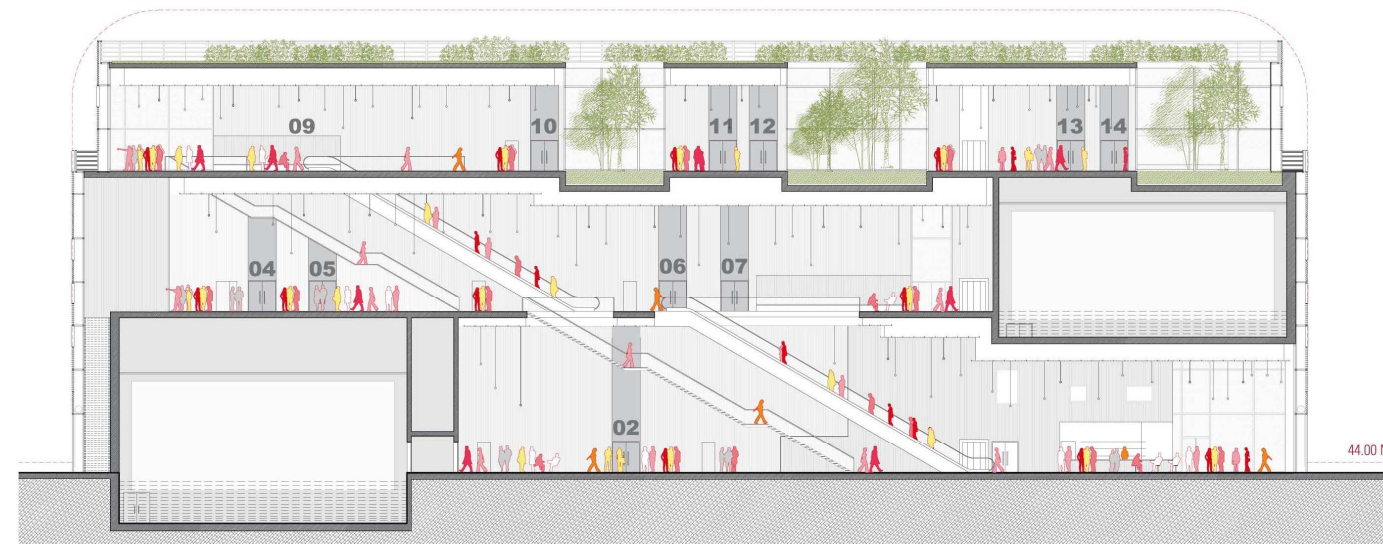
Coupe longitudinale AA', ech. : 1/200°
